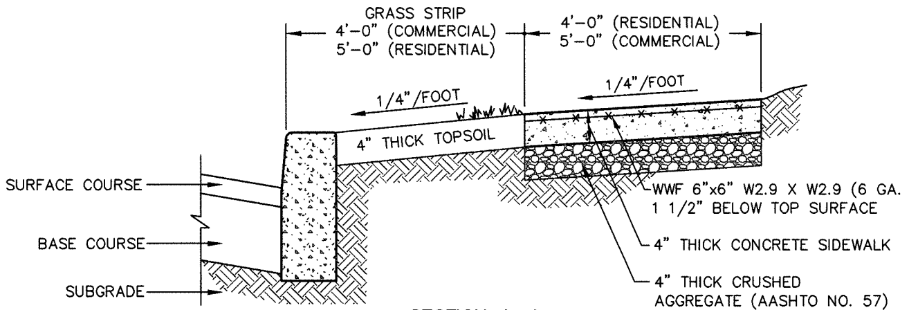
SECTION A-A
