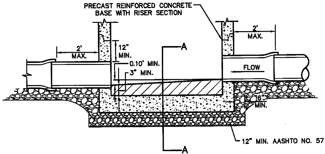
ELEVATION
